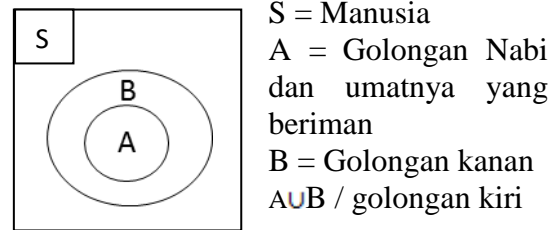
Gambar 2 venn yang digambarkan
